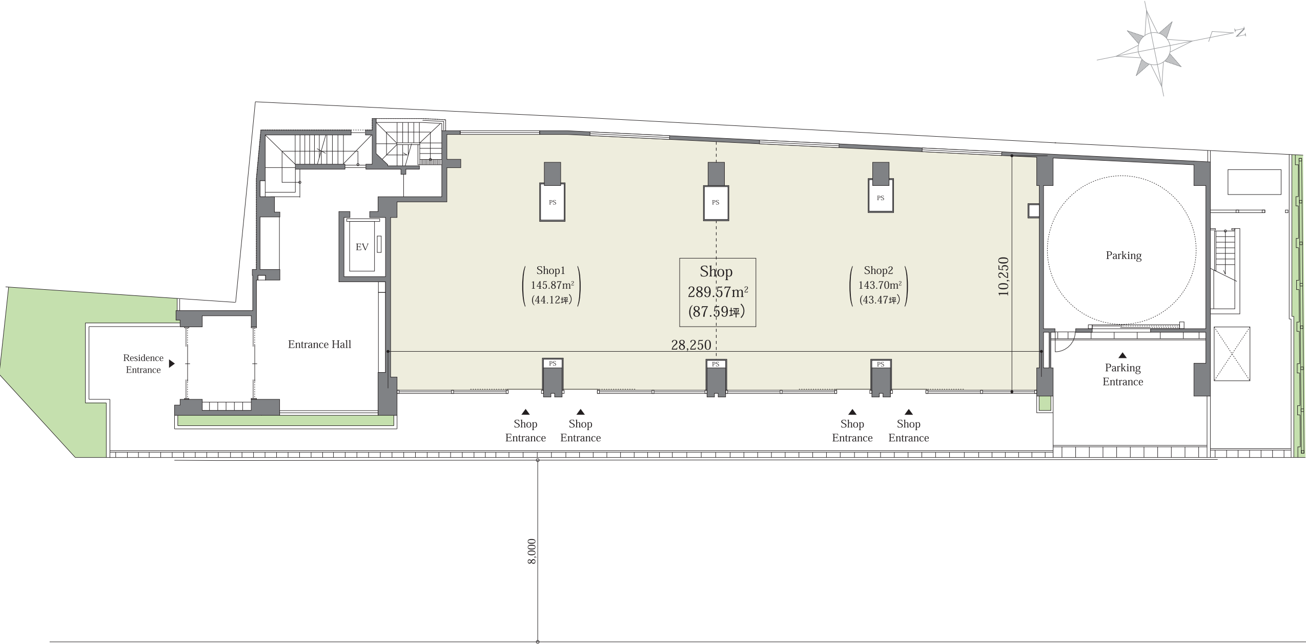
1階平面図
